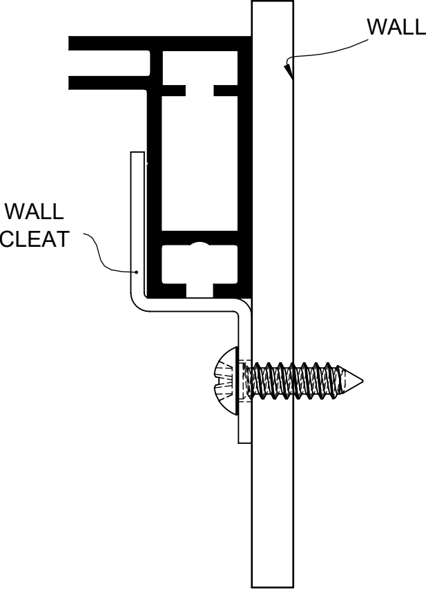
30MM SEG EXTRUSION
