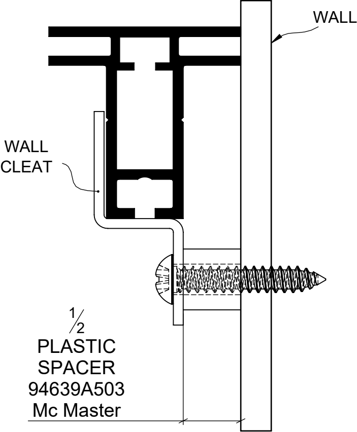
40MM SEG EXTRUSION
