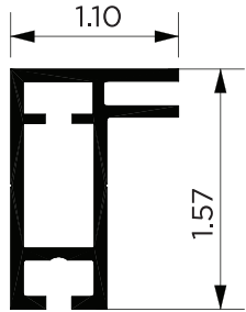
30mm SEG EXTRUSION
