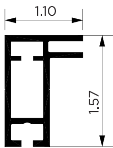
30mm SEG EXTRUSION
